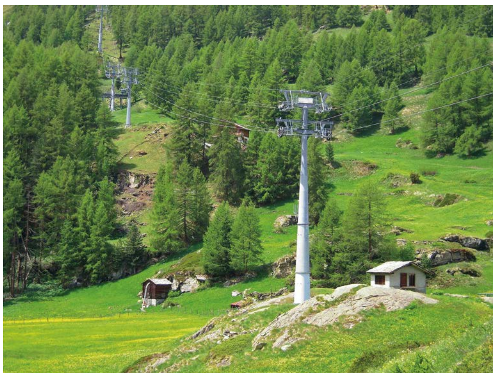
Fig. 3 > Les pylônes de télécabines présentent des dimensions généralement importantes, avec un effet marqué dans le paysage. En forêt, le tracé de l'installation nécessite des défrichements temporaires et définitifs ou des limitations de la hauteur de la forêt.
