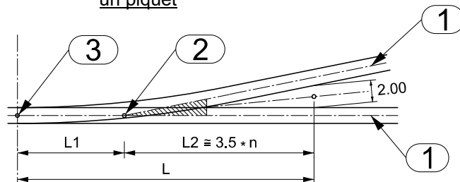
Disposition des signaux limites de garage : un piquet
