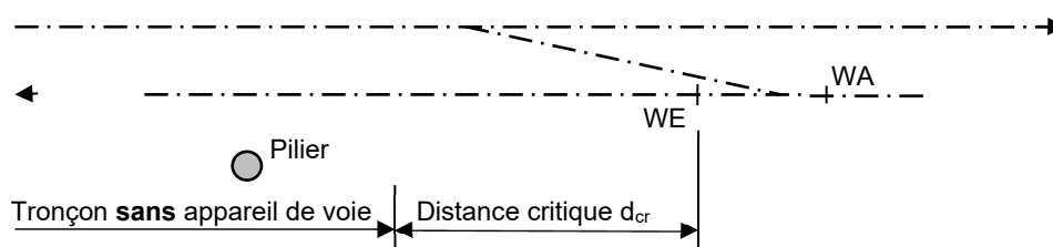
Fig. 1: Tronçon sans appareil de voie
