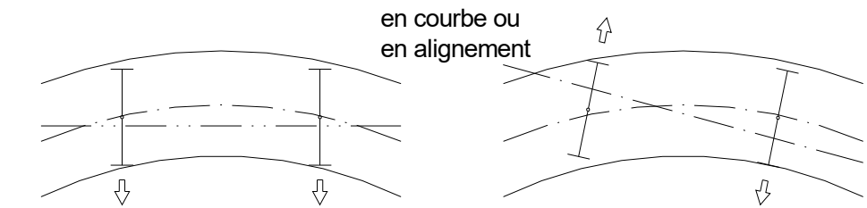
Bogies d'automotrices 1)
