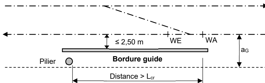
Fig. 5 : Bordure guide
