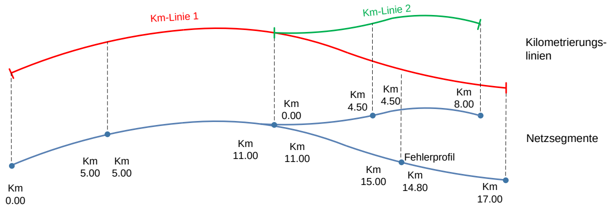
Abbildung 4: Schema Kilometrierung
