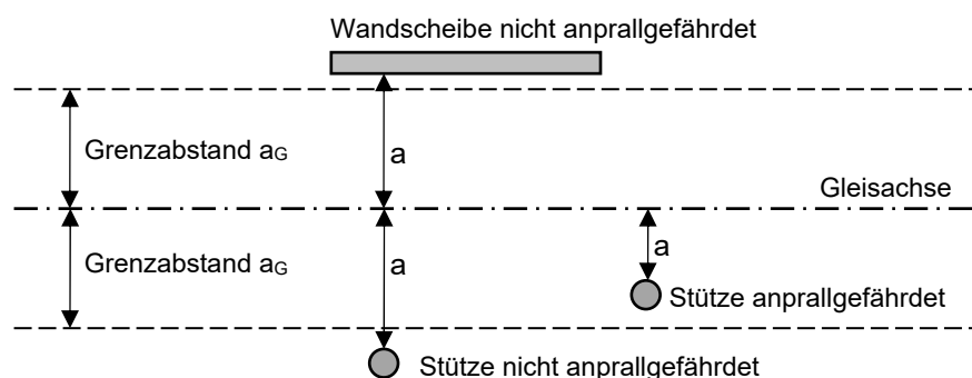
Bild 4: Grenzabstand a_G
