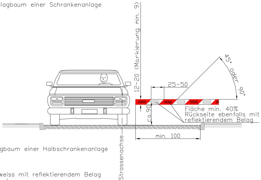
Bild 1: Schlagbäume von Schranken- und Halbschrankenanlagen
