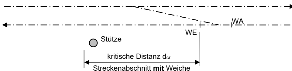
Bild 2: Streckenabschnitt mit Weiche
