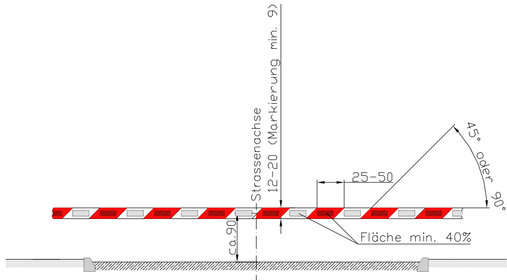
Schlagbaum einer Schrankenanlage
