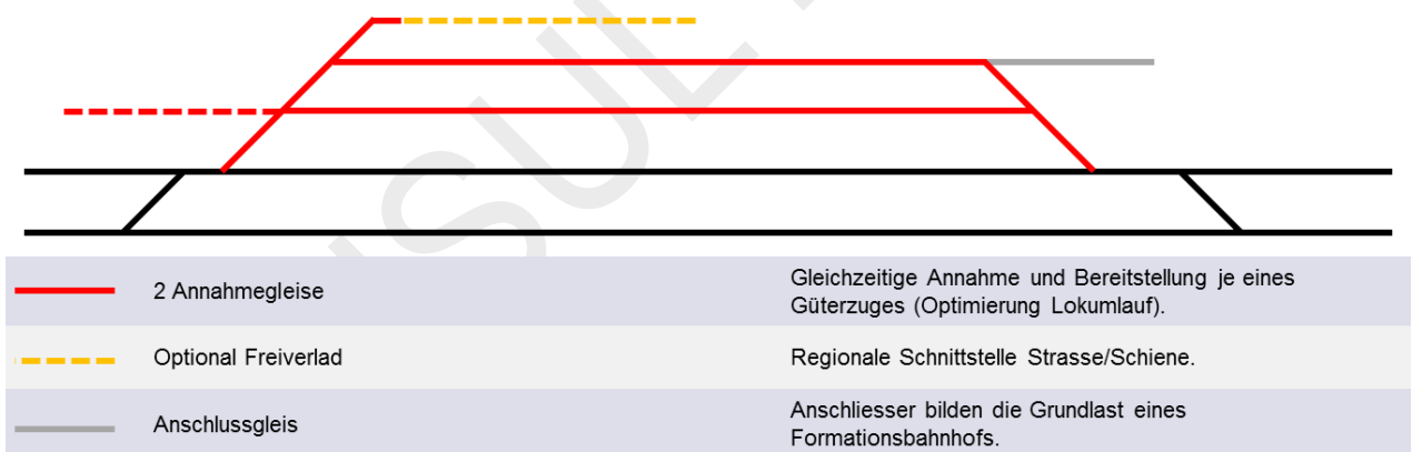
Figure 1 : structure idéale d'une gare de réception majeure
