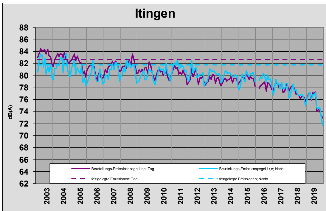
Abb. A5.2: Messstation Ittingen, Messwerte Lr,e (Monatsmittel)
