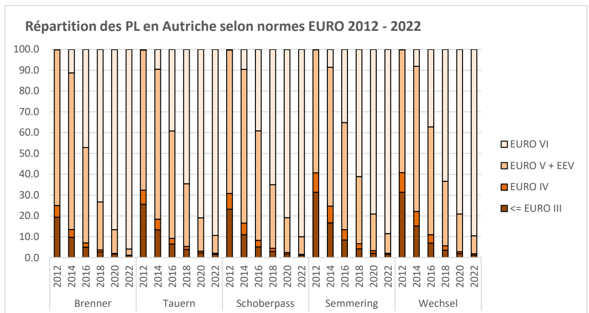
Figure 22: Répartition des poids lourds en Autriche selon normes EURO 2012 – 2022
