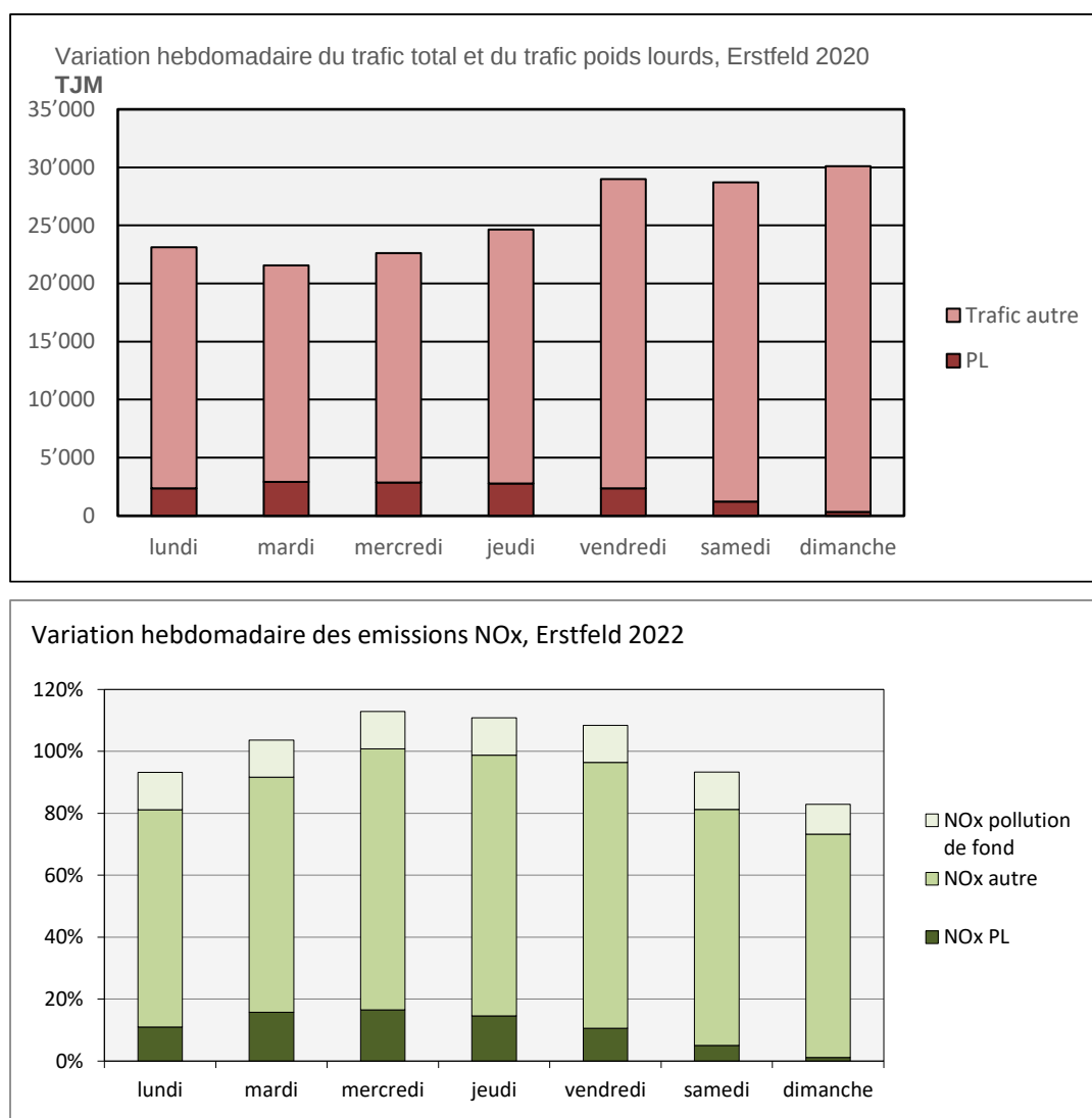
Figure 39: Variation hebdomadaire du trafic et des concentrations NO x à Erstfeld en 2020
