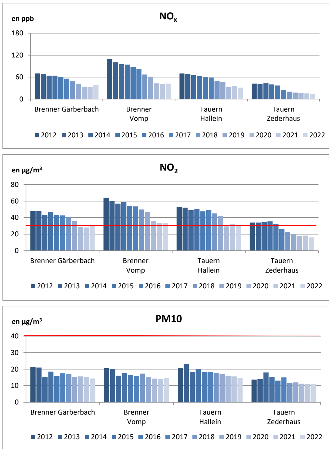
Figure 42: Concentration de \text{NO}_x , \text{NO}_2 et \text{PM}_{10} aux abords des axes autoroutiers autrichiens
